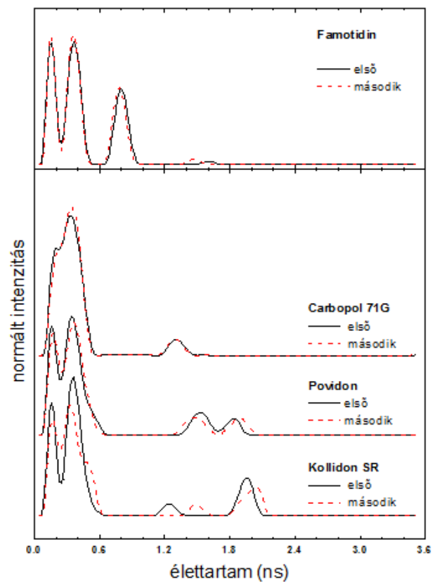
45. ábra - A referenciaminták élettartam-eloszlásai a mérősorozat elején (-) és végén (---). Az eloszlások minden esetben normáltak, hogy az intenzitások összehasonlíthatók legyenek. A b, ábrán a pozitroniumra jellemző részt emeltem ki.
