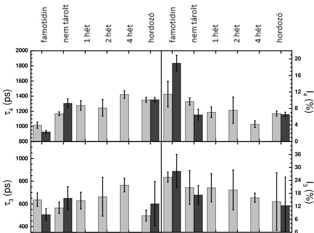
46. ábra - A famotidin-Carbopol 71G keverék öregedésének nyomon követése diszkrét kiértékeléssel. A világos oszlopok az első méréseket jelentik, a sötétek a méréssorozat végén megismételt mérések eredményét mutatják. Minden grafikonon feltüntettem a hatóanyag és a hordozó paramétereit is.
