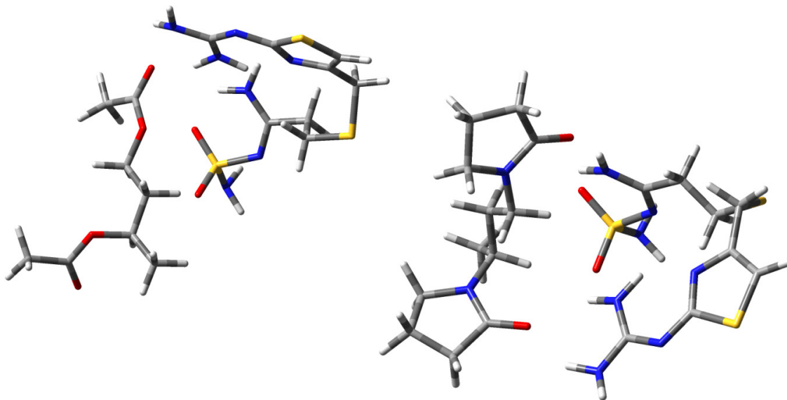
41. ábra – Famotidin – kollidon-2 dimer (N-H - - O= ) és famotidin - kollidon-1 dimer között (2 kötés: N-H - - O=) kialakuló lehetséges kötések. A famotidin – kollidon-2 komplexben a kollidon szerkezetében módosul az észterkötés.
