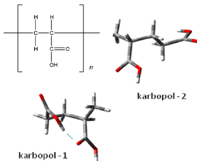
33. ábra – A Carbopol polimer szerkezete és a modellezés alapján meghatározott két dimer térbeli szerkezete. Az atomok színek: fehér - H, szürke - C, piros - O
