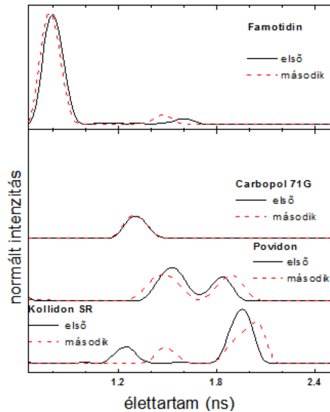
45. ábra - A referenciaminták élettartam-eloszlásai a mérősorozat elején (-) és végén (---). Az eloszlások minden esetben normáltak, hogy az intenzitások összehasonlíthatók legyenek. A b, ábrán a pozitroniumra jellemző részt emeltem ki.
