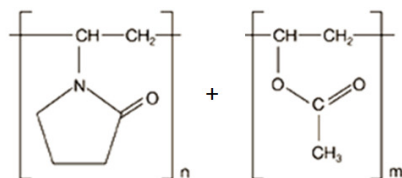
22. ábra – A Kollidon SR-t felépítő vinil-acetát és vinil-pirrolidon egységek [97]
