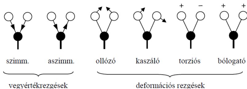
16. ábra – A metilén csoport ( =\text{CH}_2 ) vegyérték- és deformációs rezgései [68]
