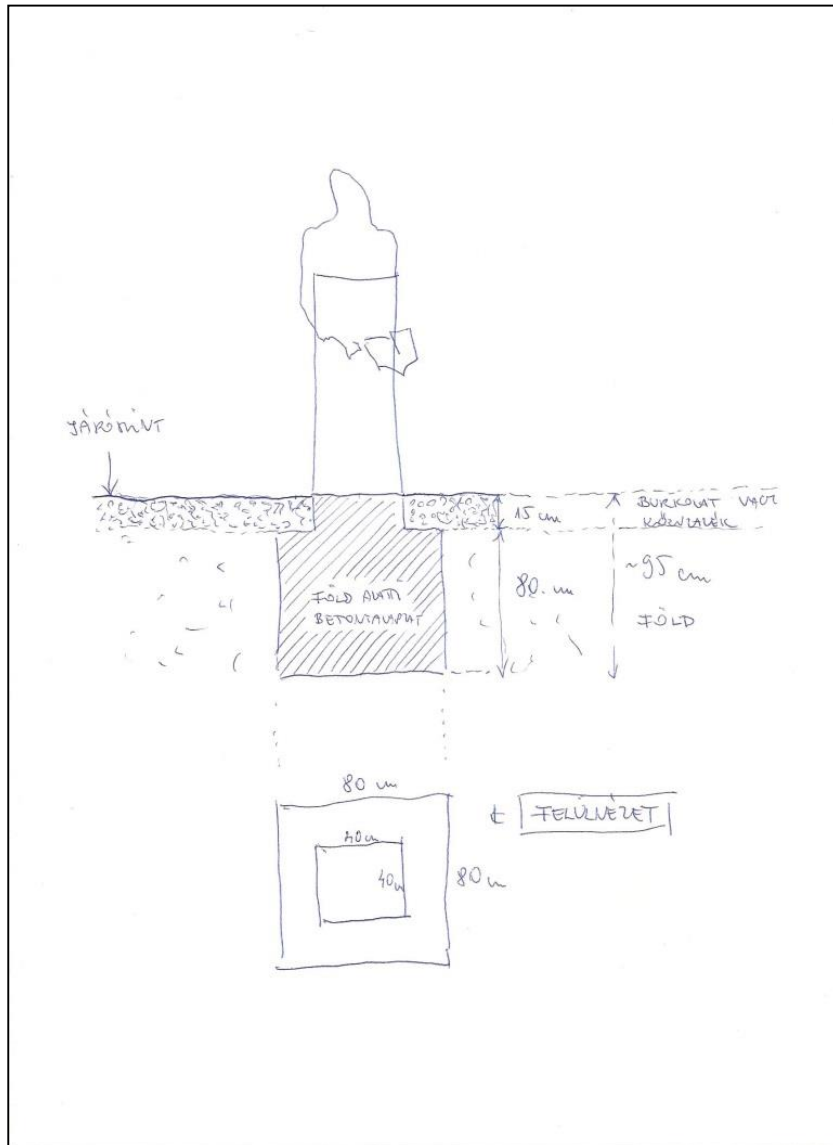
Bécsi szobor felállításához szükséges előkészítő munkák vázlata
