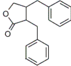
Dibenzilbutirolakton
